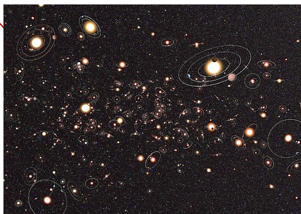
↑ 銀河系内の恒星にどのくらい惑星が存在するのかを示したイメージ図
