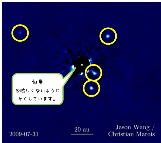
HR 8799 という恒星の周りを回る 4 つの惑星
