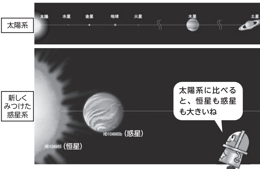
太陽系の惑星（上）と188cm反射望遠鏡で初めて発見した惑星HD104985b（下）との比較／（C）国立天文台
