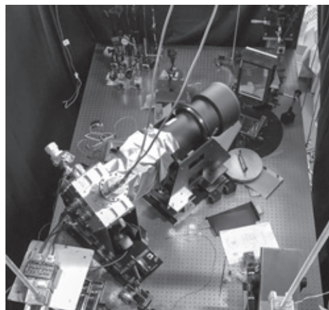
188cm反射望遠鏡にとりつけた高分散分光器。とらえた光を、さまざまな波長と強さに細かく分解することができる。／（C）国立天文台
