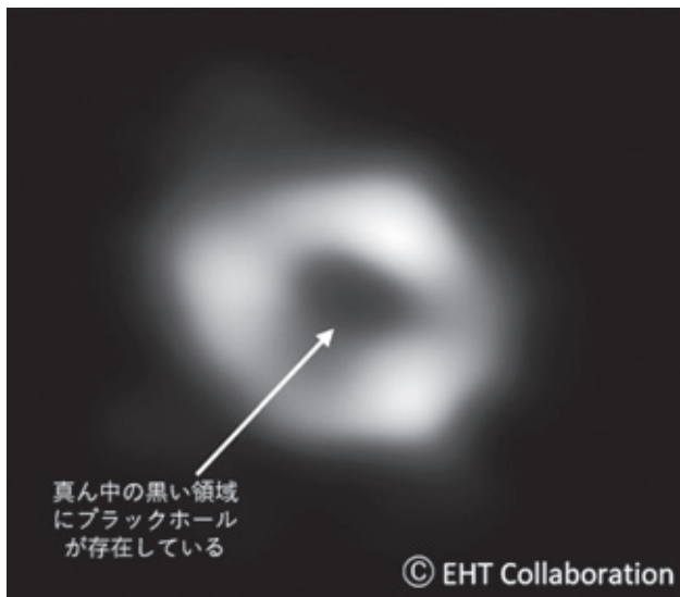
天の川銀河のブラックホール「いて座A*」
