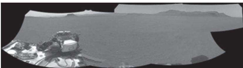
パーセバランス火星探査機により、 2022年4月14日に撮影された火星の表面。
