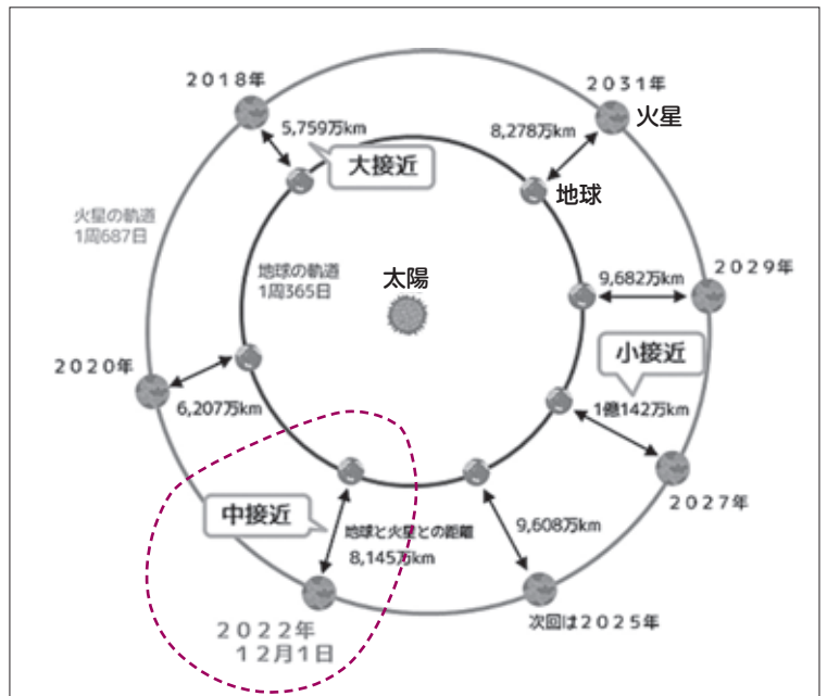
地球と火星の接近
