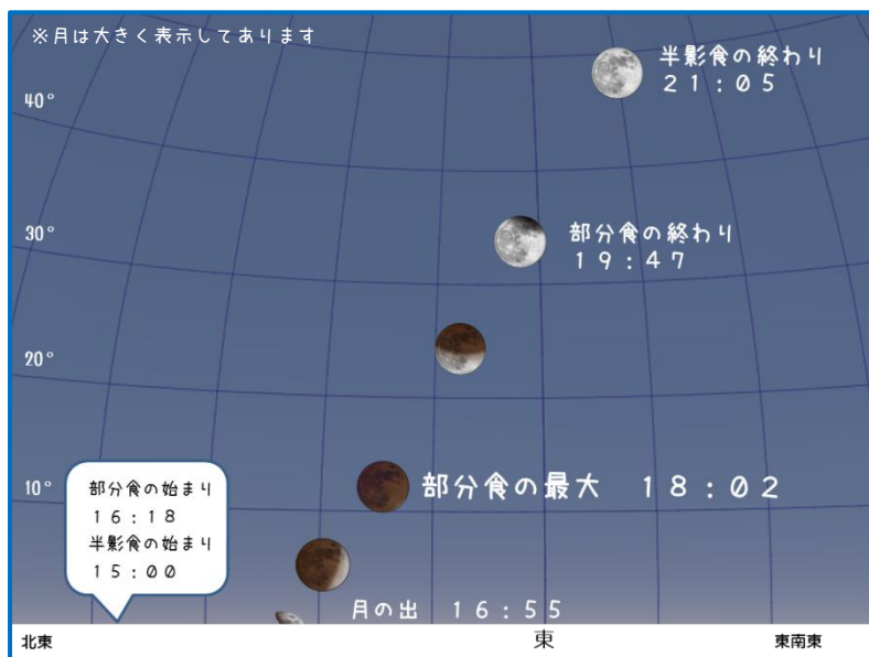
11月19日の月食の様子(ステラナビゲータで作成)
