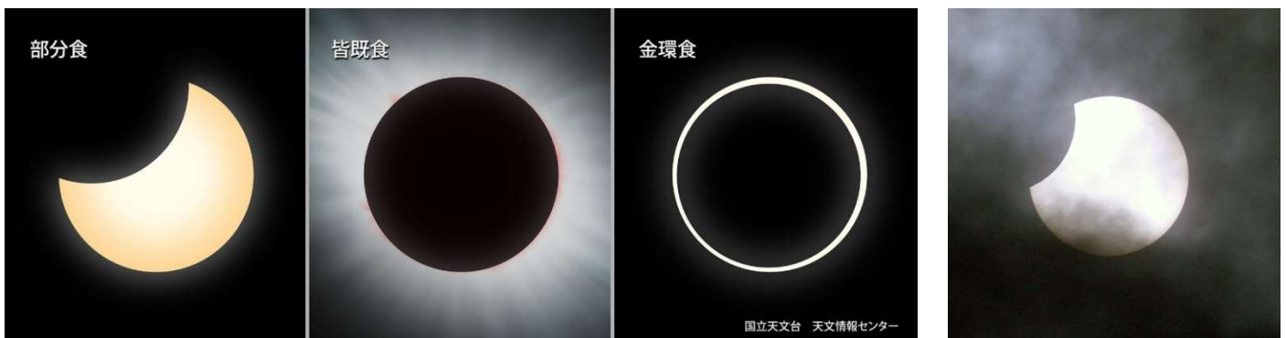
図. 日食の種類（提供：国立天文台 天文情報センター）
