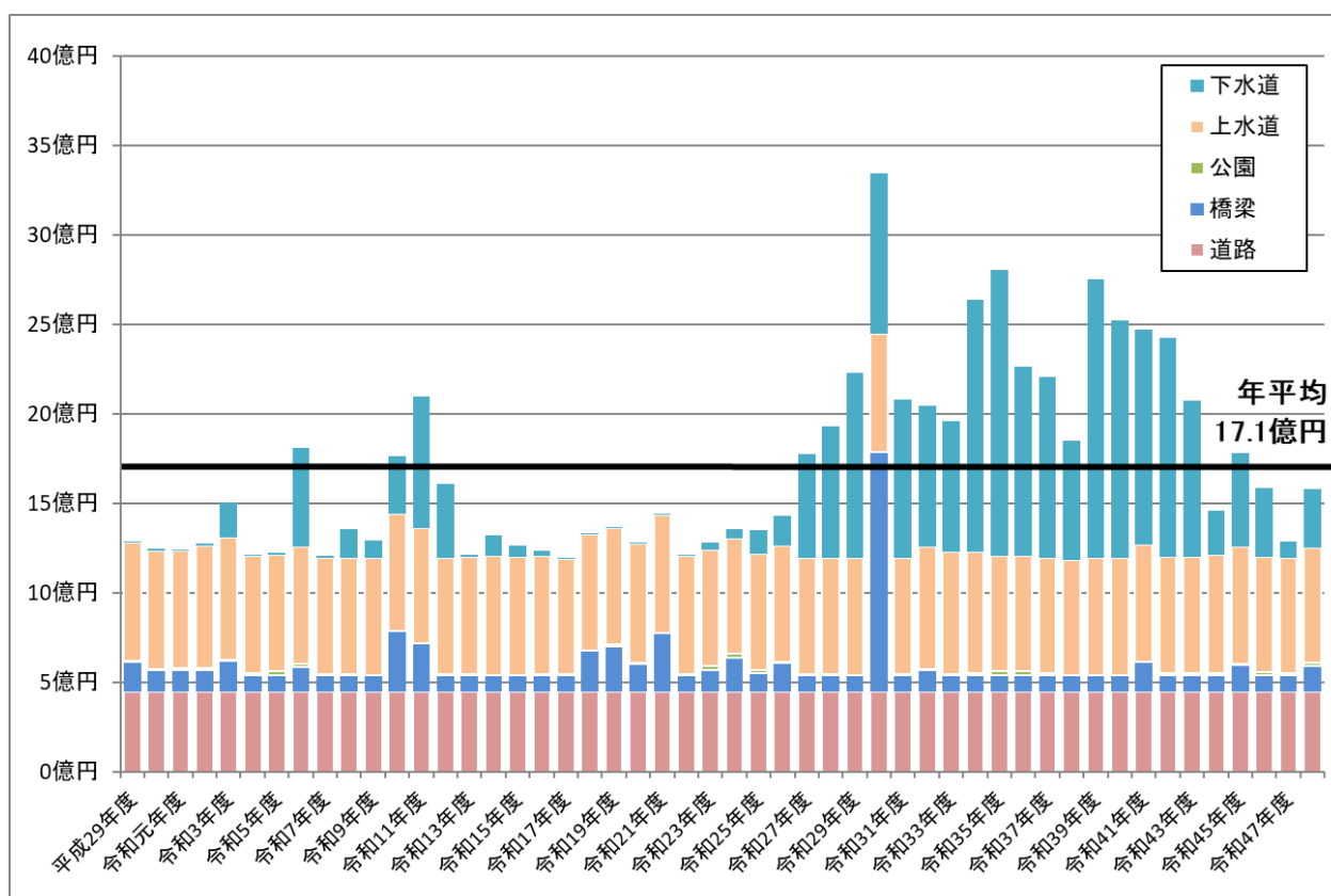
図 4-2 インフラ施設の将来更新費用
